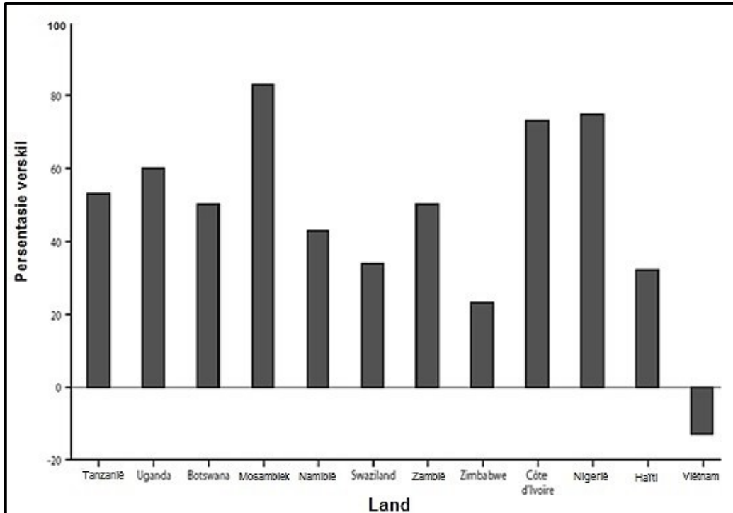
FIGUUR 3.5: OORSTROMINGS
