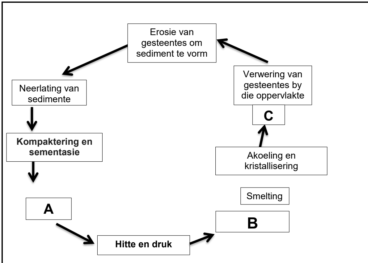
FIGUUR 1.5: GESTEENTESIKLUS
